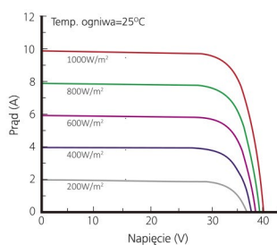
Wykres prąd-napięcie
