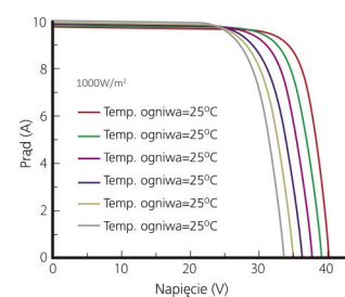
Wykres prąd-napięcie
