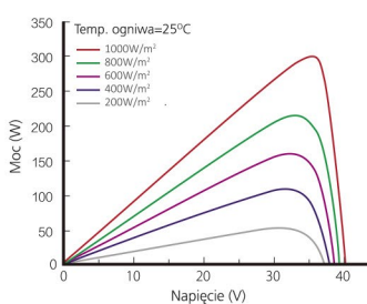
Wykres moc-napięcie
